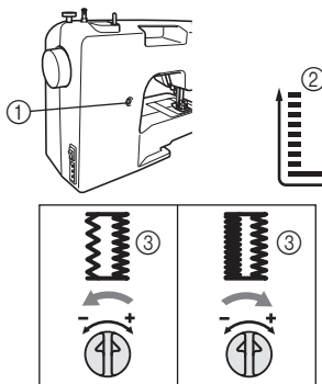
1 Винт точной настройки обметывания петель 2 Левая сторона 3 Вид петли
